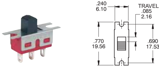
SPDT
